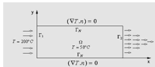
FIG. 1 – Température ( 200^\circ\text{C} ) et vitesse imposées
