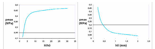
Fig. 9. p_{max} as a function of H/h_0 : h_0=0,25\text{mm} and h_0 : H/h_0=4 - R=125\text{mm} ; U=1,5\text{m/min} ; K=3000\text{Pa.s}^m ; m=0,62
