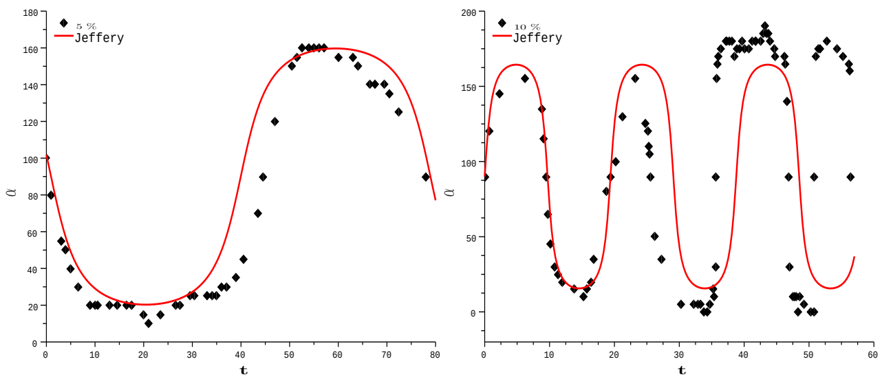
FIG. 3 – Mesures de l'angle \alpha pour les deux concentrations \Phi_s = 5 et 10 % ; les courbes rouges (ou continues) correspondent à la solution de Jeffery.
