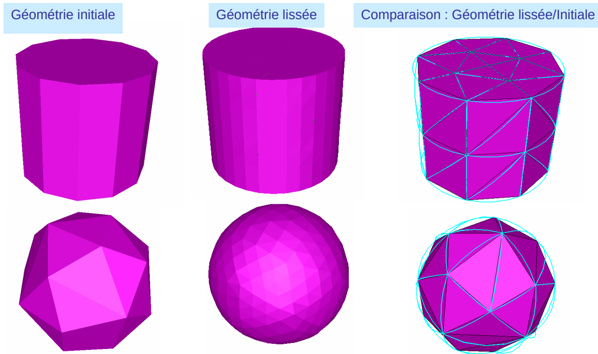
FIG. 11 – Effet de l'interpolation C2 pour une sphère et un cylindre
