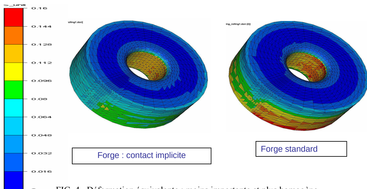
FIG. 4– Déformation équivalente : moins importante et plus homogène
