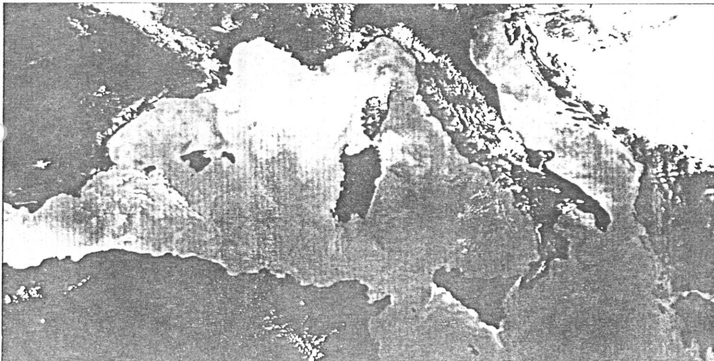
Thermographie de la Méditerranée Occidentale d'après le satellite TIROS-N :
